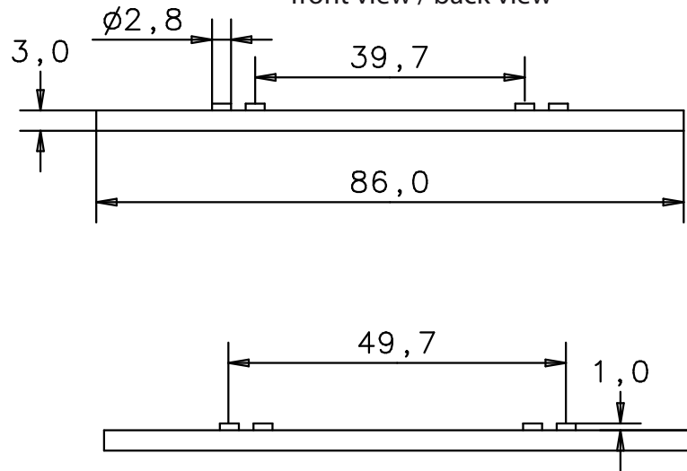
Vorderansicht / Rückansicht front view / back view
