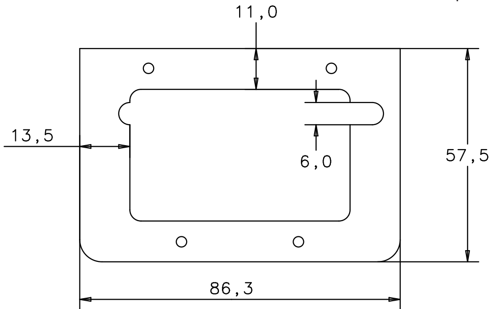
Draufsicht / Untersicht top view / bottom view
